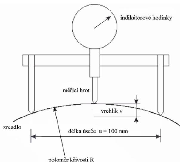
Obr. 4: Schéma měření poloměru křivosti zrcadla
