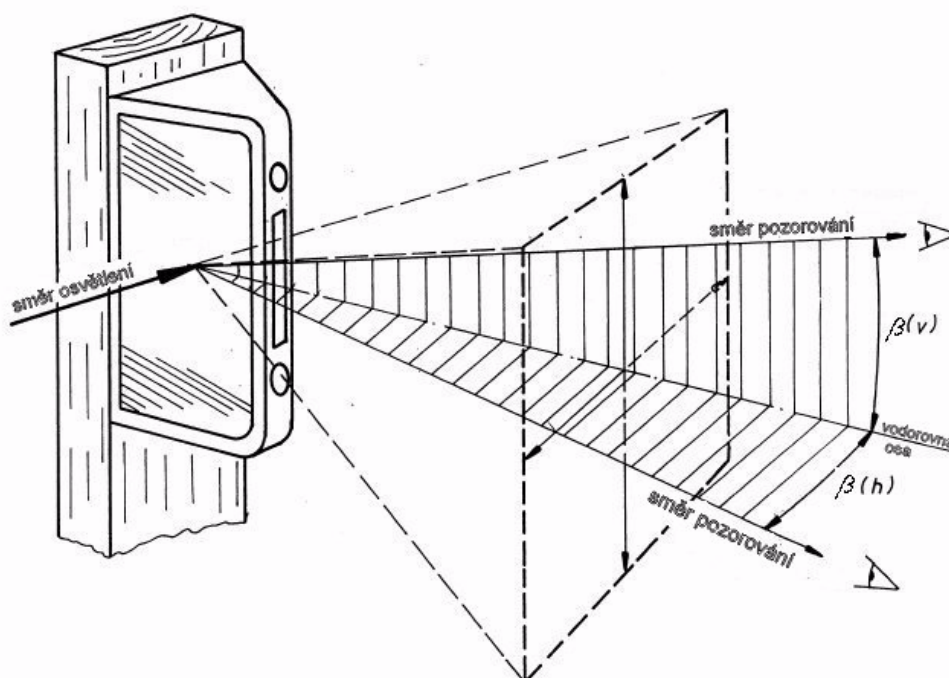
Obr. 13: Schéma pozorovacích úhlů
