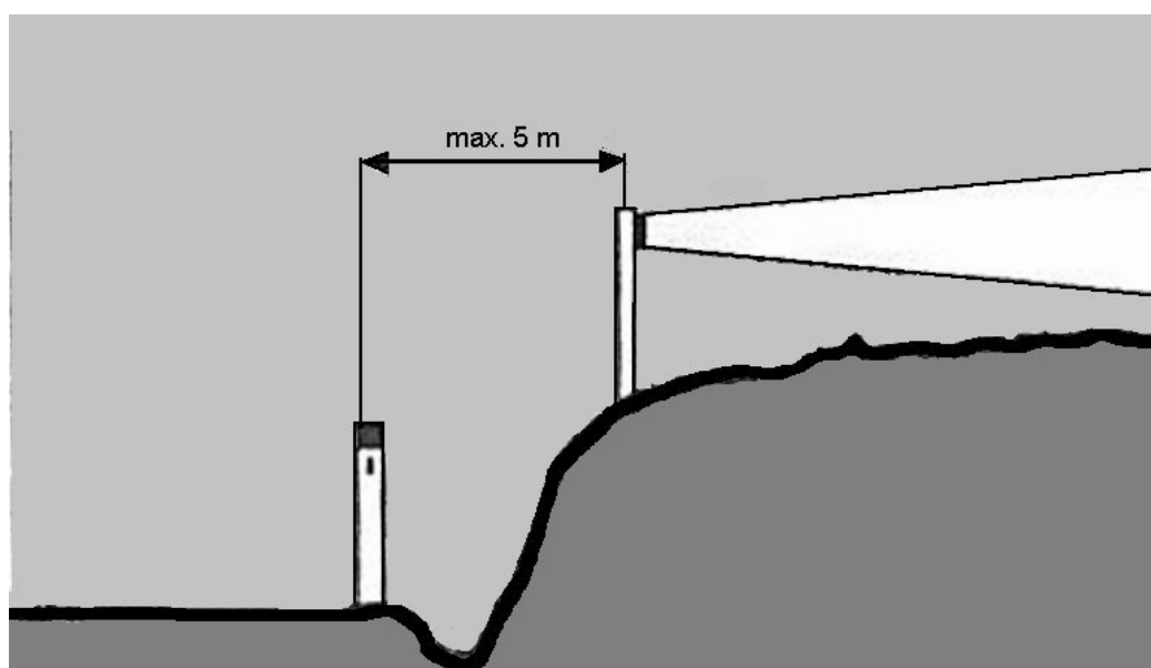
Obr. 9: Umístění odražeče mimo komunikaci
