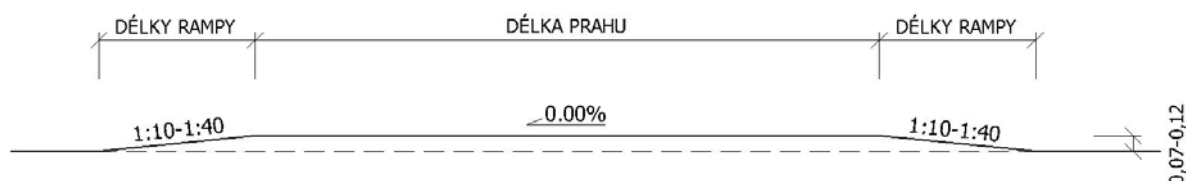
Obrázek 11 - Lichoběžníkový tvar zpomalovacího prahu
