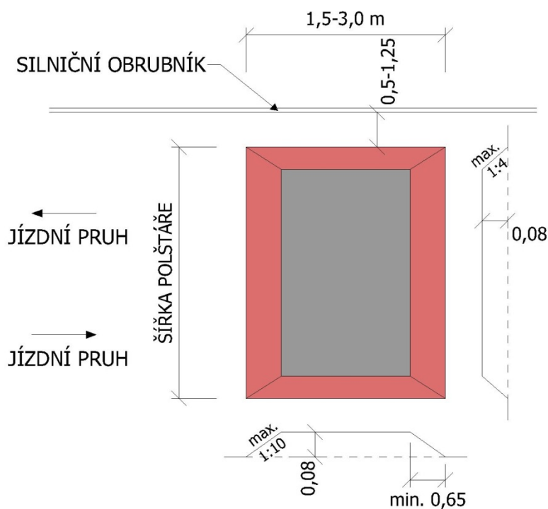
Obrázek 18 - Lichoběžníkový tvar zpomalovacího polštáře přes více jízdních pruhů
