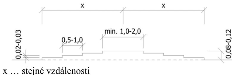
Obrázek 12 - Stupňovitý tvar zpomalovacího prahu
