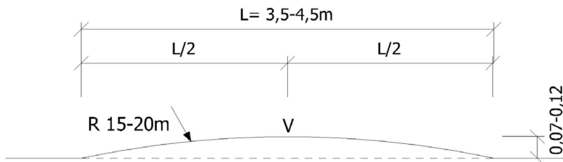
Obrázek 14 - Kruhový tvar zpomalovacího prahu
