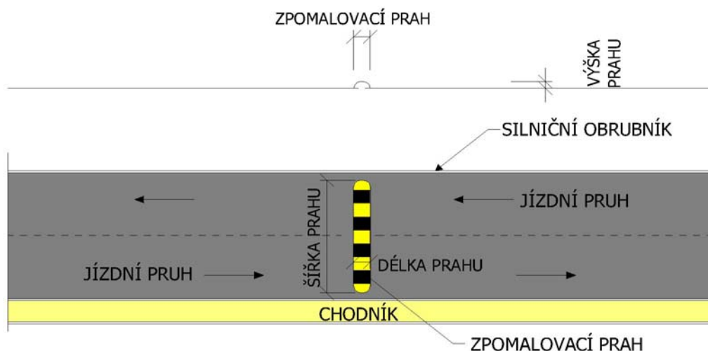
Obrázek 1 - Krátký zpomalovací prah
