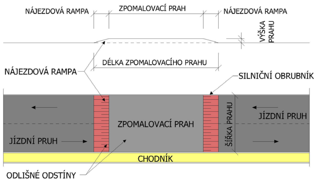
Obrázek 2 - Dlouhý zpomalovací práh prostý
