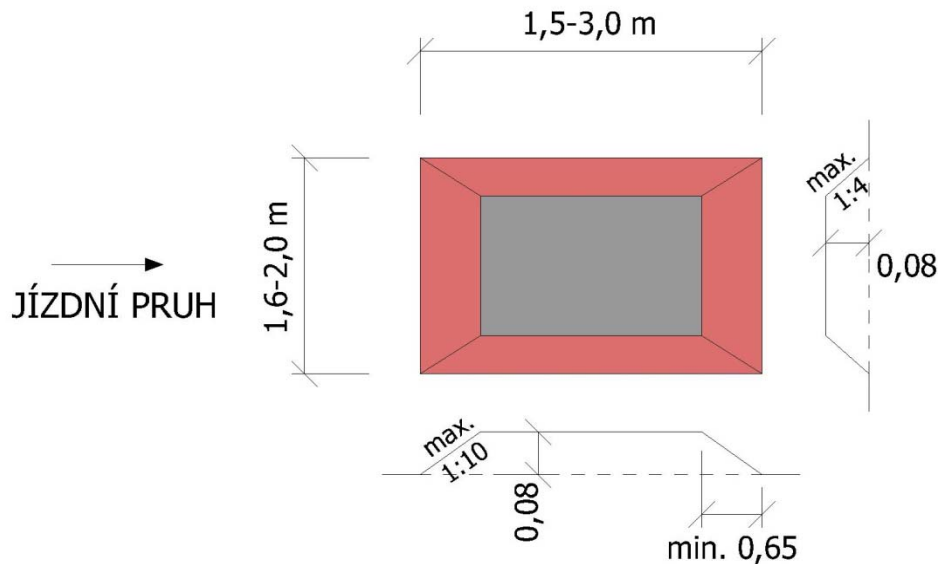
Obrázek 17 - Lichoběžníkový tvar zpomalovacího polštáře v jednom jízdním pruhu
