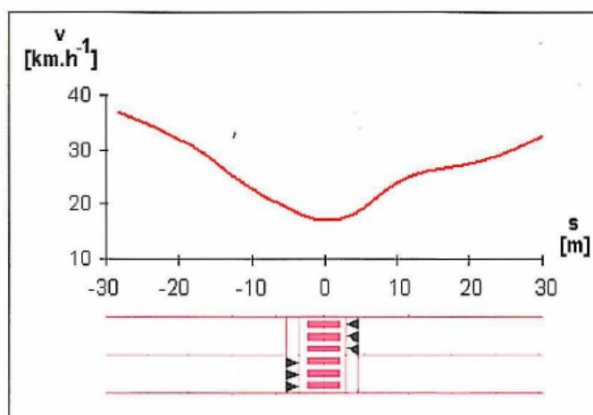
Obrázek 9 - Příklad účinku snížení rychlostí vozidel při užití dlouhého zpomalovacího prahu konstruovaného na rychlost 20 km.h -1 .
