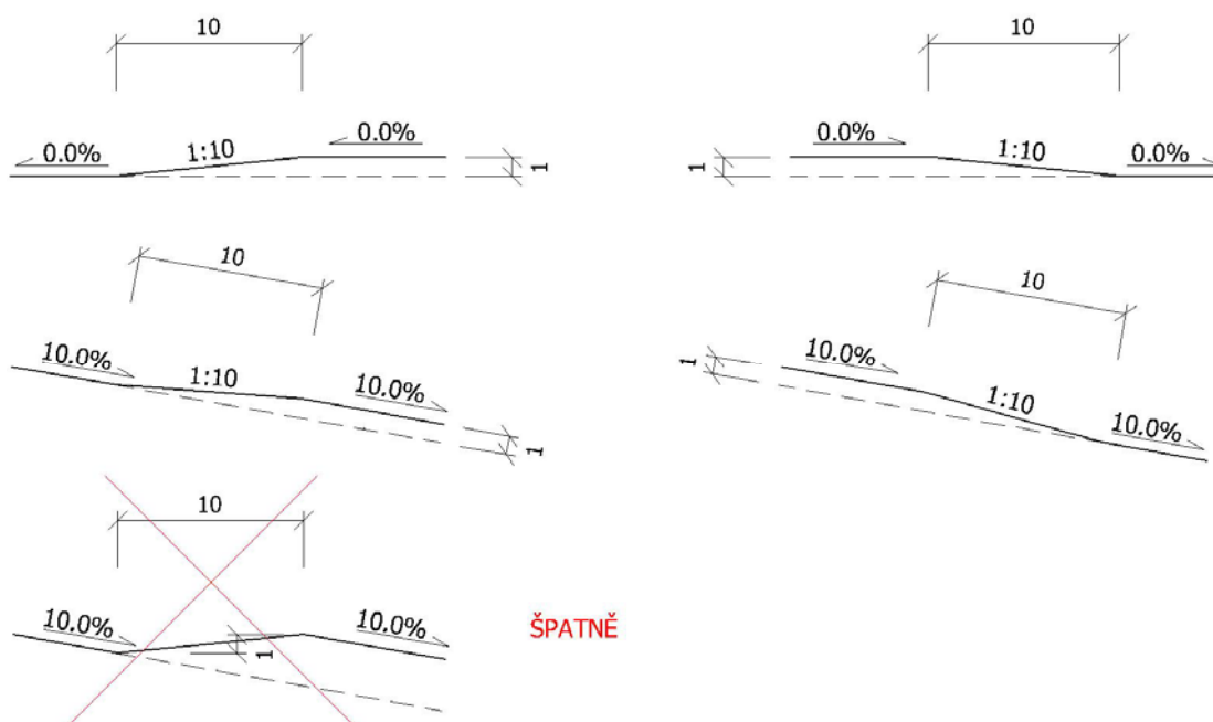
Obrázek 10 - Příklad sklonu nájezdové rampy v závislosti na sklonu nivelety
