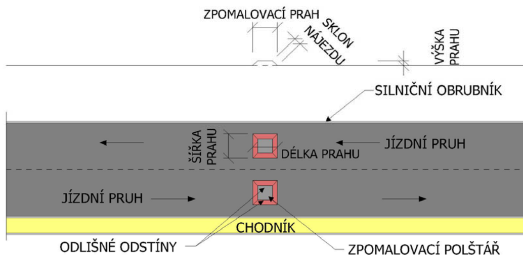
Obrázek 3 - Zpomalovací polštář
